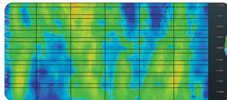
储罐分析
